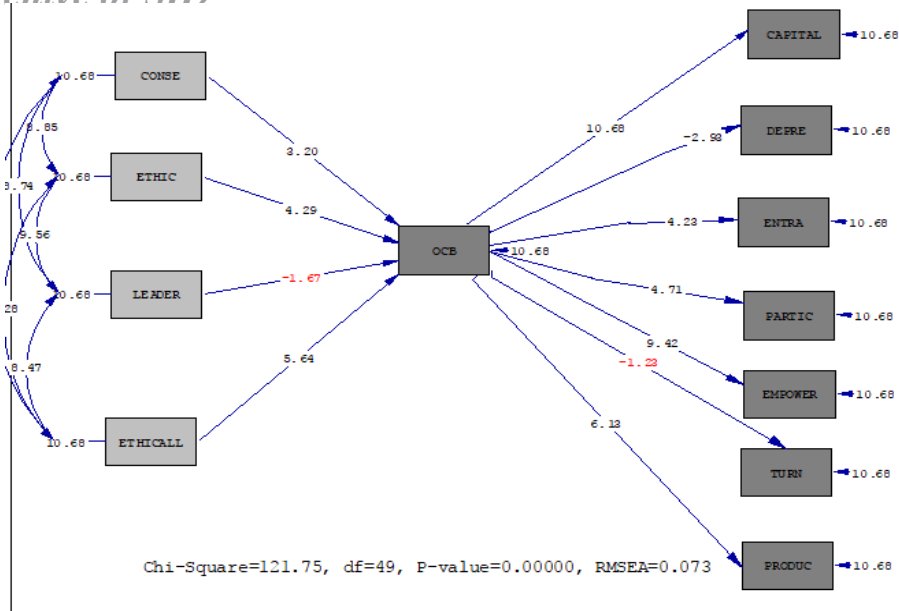
شکل ۳: خروجی نرم افزار بر اساس ضرایب t
