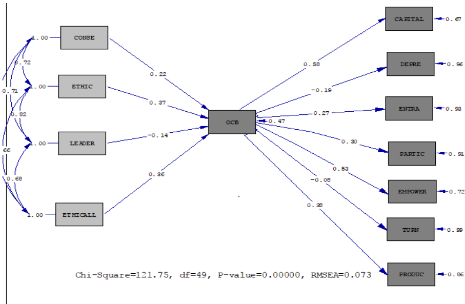
شکل ۲: خروجی نرم افزار بر اساس ضرایب استاندارد
