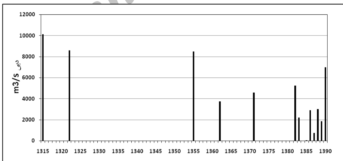
شکل ۱۵ نمودار دبی سیلاب های جدید و قدیمی (بازسازی شده)
