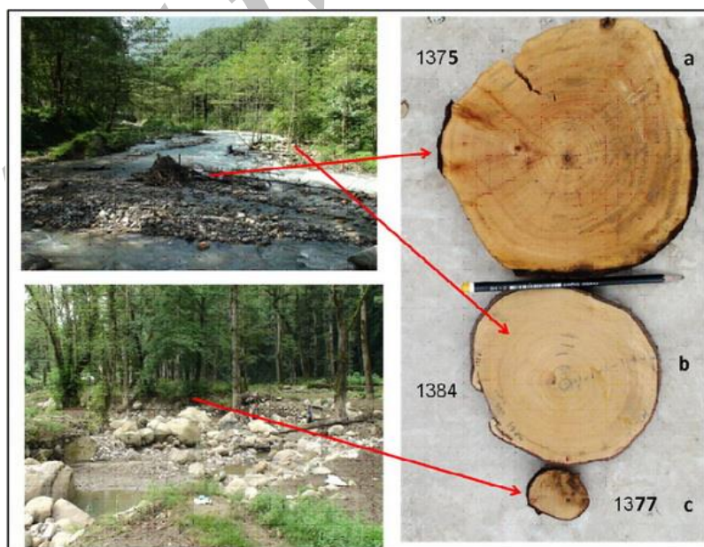
شکل ۶ مقاطع عرضی از تنه درختان حاشیه بستر اصلی (a,b) و بسترهای فرعی (c)
