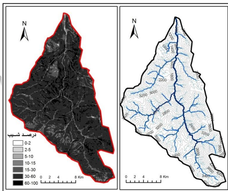
شکل ۲ توپوگرافی و شیب در حوضه آبریز سه هزار
