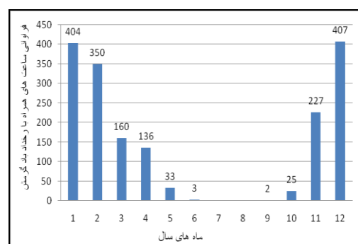
شکل ۳ مجموع فراوانی ساعتی وقوع باد گرمش در ماه های مختلف سال (۲۰۱۰-۱۹۸۲)
