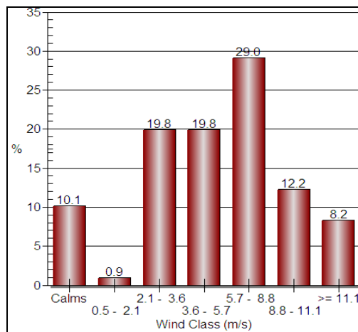
شکل ۸ توزیع فراوانی دسته های مختلف سرعت باد در زمان وزش باد گرمش ایستگاه همدیدی رشت (۱۹۸۲-۲۰۱۰)
