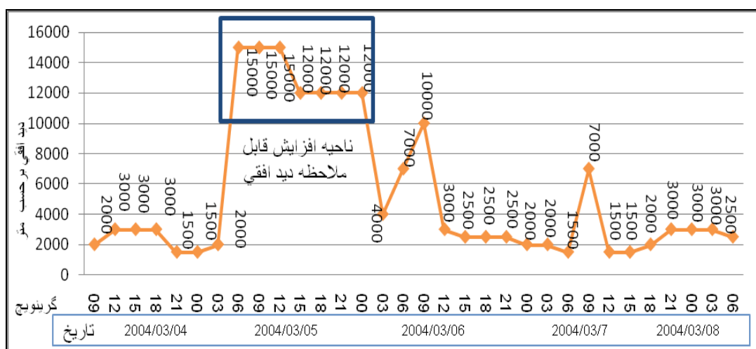
شکل ۱۶ افزایش شدید دید افقی در طول زمان رخداد باد گرمش در ایستگاه همدیدی رشت
