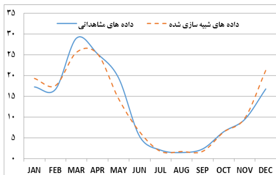
شکل ۱۲ شبیه‌سازی بارش در ایستگاه شاهرود در سناریوی
