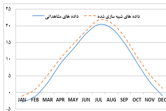
شکل ۱۴ شبیه‌سازی دمای کمینه در ایستگاه شاهرود
