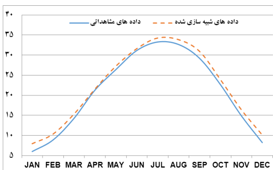
شکل ۱۸ شبیه‌سازی دمای بیشینه در ایستگاه شاهرود در سناریوی A2
