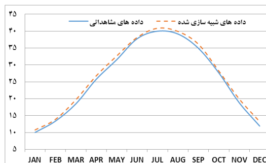
شکل ۲۷ شبیه‌سازی دمای بیشینه در ایستگاه گرمسار در سناریوی B1
