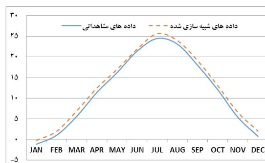
شکل ۲۳ شبیه‌سازی دمای کمینه در ایستگاه گرمسار
