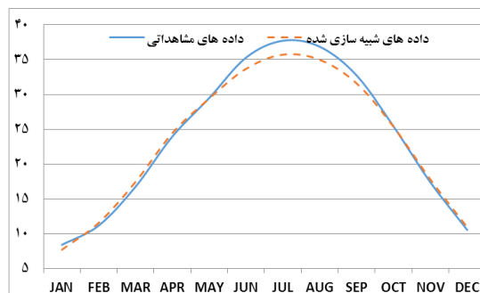
شکل ۳۶ شبیه‌سازی دمای بیشینه در ایستگاه سمنان در
