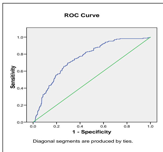
شکل ۶ منحنی ROC
