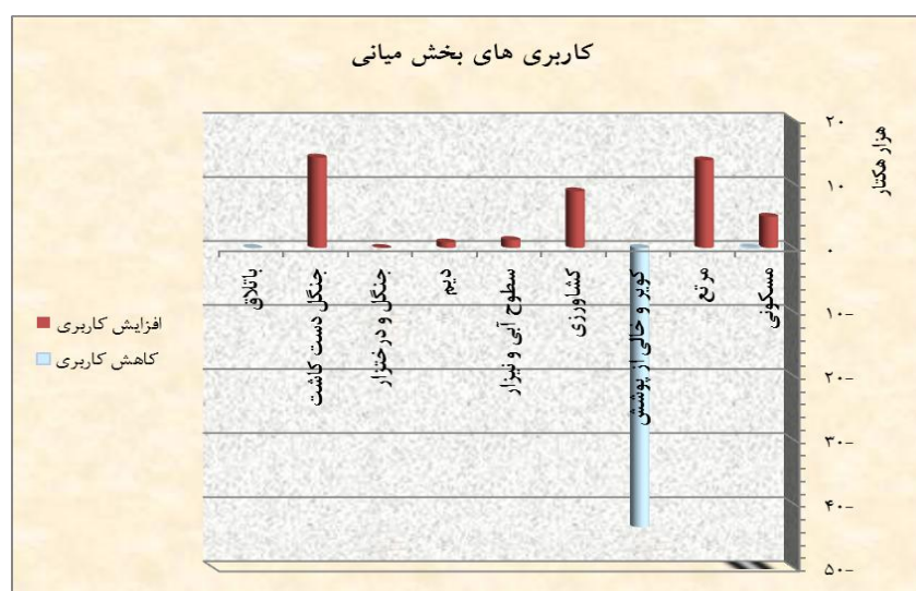
شکل ۶ تغییرات کاربری زمین در قسمت میانی حوضه آبریز زاینده‌رود (۲۰۱۳-۲۰۰۲)
