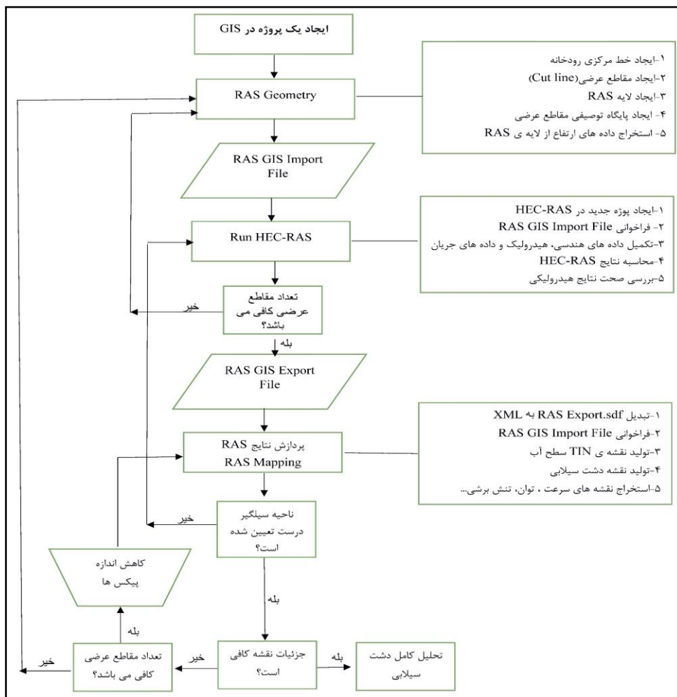
شکل ۲. روند شبیه‌سازی سیلاب با استفاده از الحاقی HEC-GeoRAS و مدل هیدرودینامیکی HEC-RAS (Cameron, 2009)
