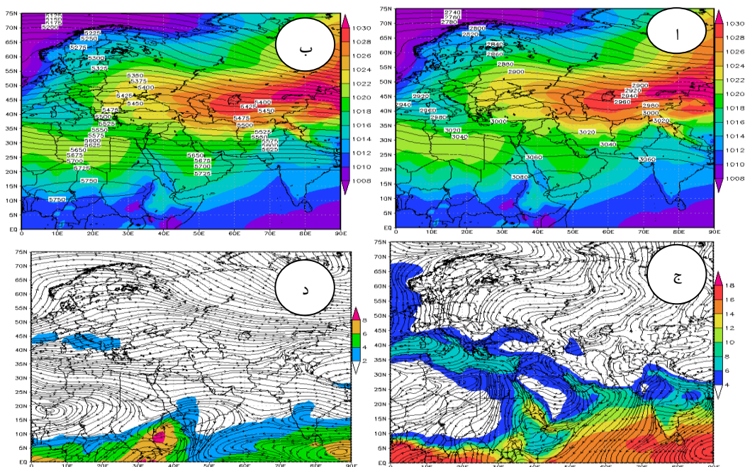
شکل ۳- نقشه ترکیبی فشار تراز دریا و ارتفاع ژئوپتانسیل در تراز الف: ۷۰۰ و ب: ۵۰۰ هکتوپاسکال، نقشه ترکیبی بردار باد و رطوبت در تراز ج: ۱۰۰۰ و د: ۷۰۰ هکتوپاسکال میانگین ژانویه تا مارس ۲۰۰۱
