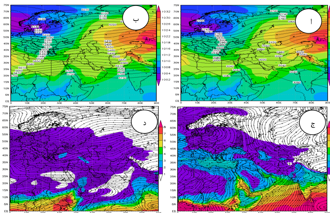
شکل ۷- نقشه ترکیبی فشار تراز دریا و ارتفاع ژئوپتانسیل در تراز الف: ۷۰۰ و ب: ۵۰۰ هکتوپاسکال، نقشه ترکیبی بردار باد و رطوبت در تراز ج: ۱۰۰۰ و د: ۷۰۰ هکتوپاسکال میانگین ژانویه تا آوریل و دسامبر ۱۹۸۶
