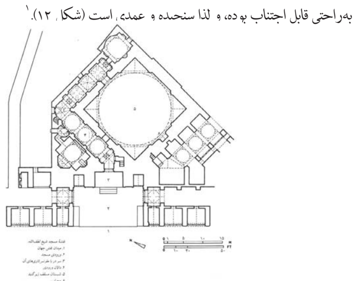
شکل ۱۲. پلان مسجد شیخ لطف الله
