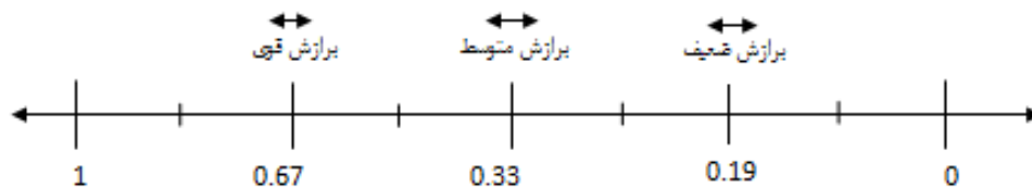
شکل ۳: چگونگی سنجش برازش بخش ساختاری مدل به وسیله R^2
