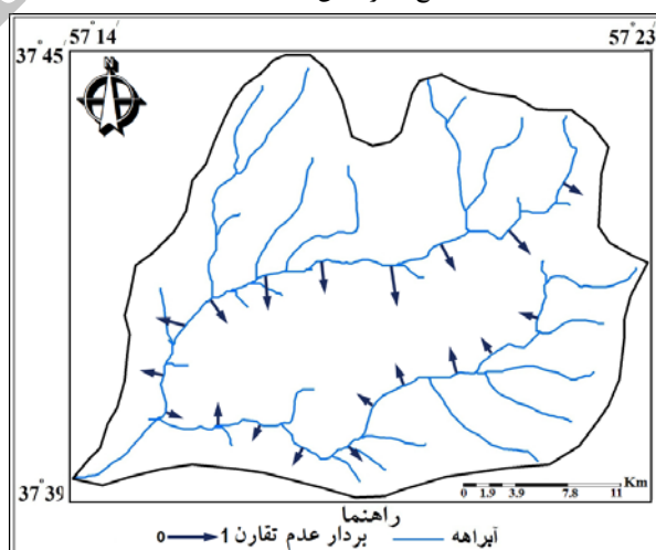
شکل ۸: ارزیابی شاخص فاکتور تقارن توپوگرافی معکوس (T) در حوضه اصلی
