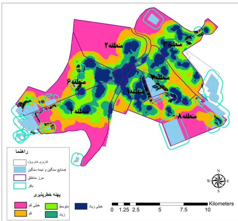
نقشه ۶. شعاع تخریب و چگونگی توزیع مکانی صنایع سنگین و نیمه‌سنگین در مناطق هفت‌گانه شهر اهواز (منبع: نگارندگان، ۱۳۹۵)
