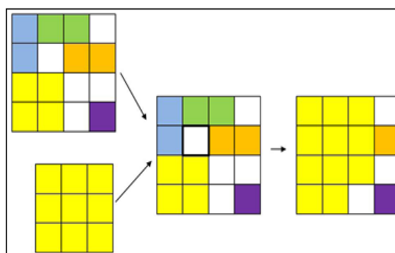
شکل ۶. عملگر جهش
