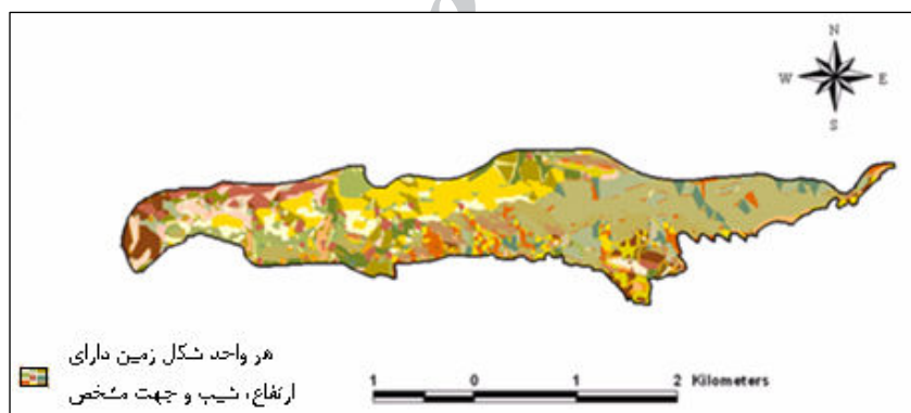
شکل ۵. نقشه واحدهای شکل زمین پارک جنگلی سرخه‌حصار
