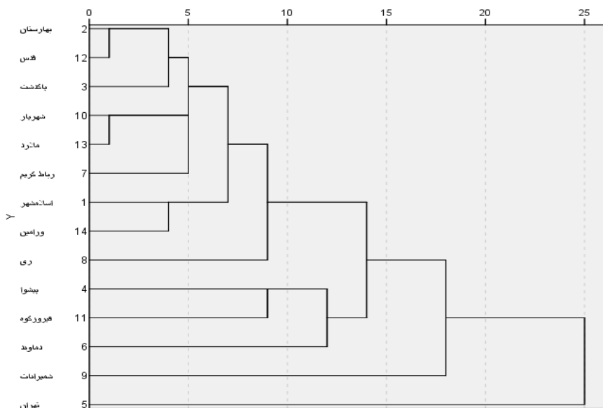
شکل ۵. نمودار درختی
