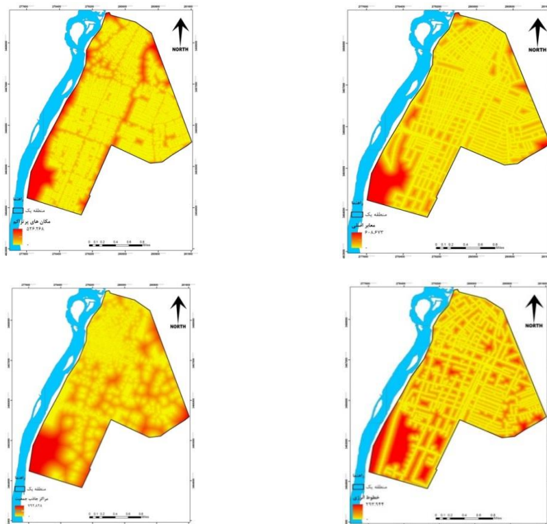
نقشه ۲. فاصله از مکان‌های پرتراکم، فاصله از مراکز جاذب جمعیت، فاصله از معابر اصلی جهت دسترسی و جابه‌جایی، فاصله از خطوط انرژی در منطقه مورد مطالعه
