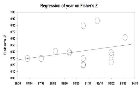
شکل ۲- نتایج متارگرسیون برای هر یک از مطالعات
