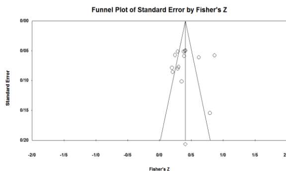
شکل ۱- نمودار کیفی برای بررسی خطای انتشار
