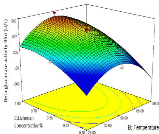
شکل ۴- نمودار سه بعدی اثر متقابل دما و غلظت سوستر بر فعالیت بتاگلوکاناز باسیلوس ساتیلیس B5d در نقطه مرکزی اسیدیته
