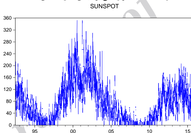
شکل ۳- تعداد نقاط تاریک روی سطح خورشید در یک روز (بر مبنای سال میلادی) ۱۴
