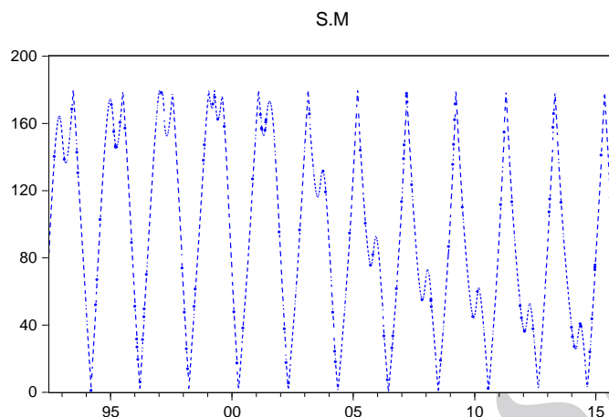
شکل ۲- داده‌های مرتبط با زاویه (درجه) مابین موقعیت زحل و مریخ (از دید مشاهده‌گر زمینی بر مبنای سال میلادی).
