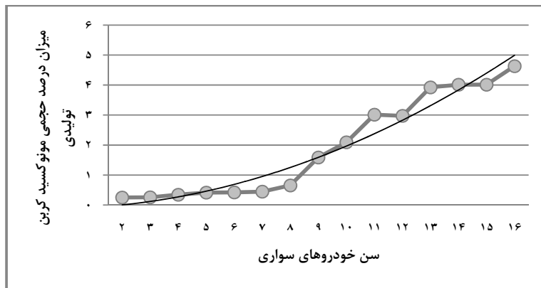
نمودار ۵- رابطه بین سن و درصد حجمی مونواکسید کربن تولیدی خودروهای سواری (مطالعات نگارندگان)
