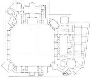
▲ نقشه ۲. پلان طبقه هم‌کف حسینی‌ی نواب (صابر مقدم، بی‌تا).
