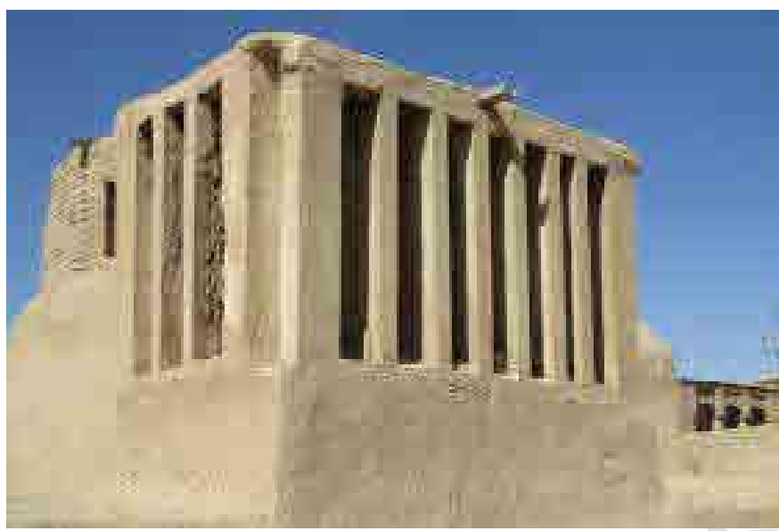
تصویر ۹. نمای بادگیر چهارطرفه حسینی‌نواب (نگارندگان، ۱۳۹۳).
