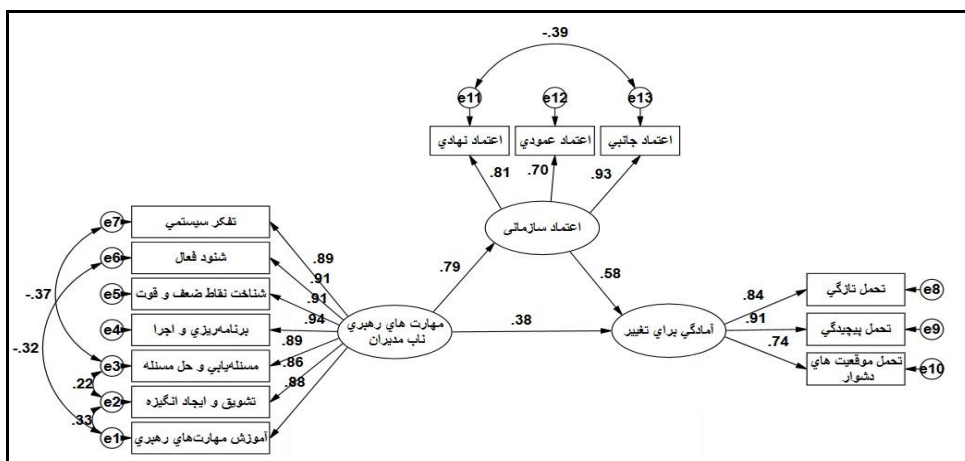
شکل ۲. الگوی آموس در حالت تخمین استاندارد
