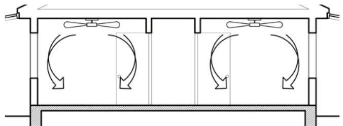
نگاره (۳): طرح شماتیک فن سقفی پیشنهادی برای خانه نمونه طراحی اقلیمی برای تهران
