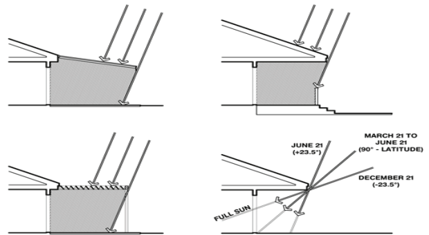
نگاره (۲): تصویر شماتیک سایبان‌های پیشنهادی برای خانه نمونه طراحی اقلیمی برای تهران
