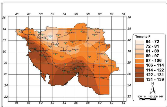
نگاره (۶): نقشه پهنه‌بندی دمای احساس بلندمدت ژوئن
