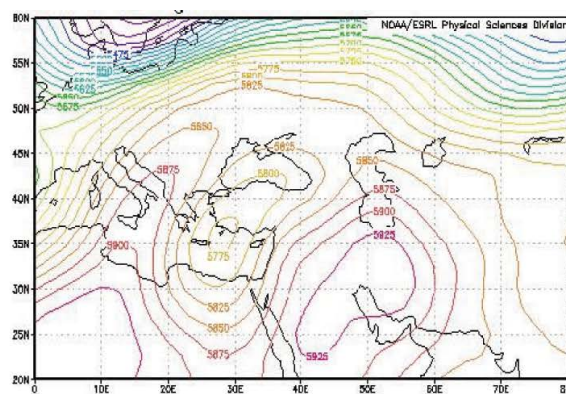
نگاره (۱۱): الگوی سینوپتیکی حاکم در تراز ۵۰۰ هکتوپاسکال در روز ۱۳۸۹/۴/۲۲
