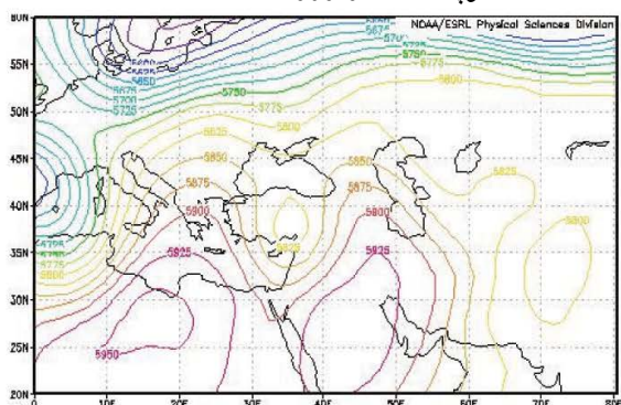
نگاره (۱۴): الگوی سینوپتیکی حاکم در تراز ۵۰۰ هکتوپاسکال در روز ۱۳۸۹/۴/۲۵
