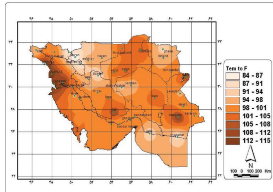
نگاره (۳): نقشه پهنه‌بندی دمای بلندمدت ژوئن
