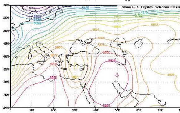
نگاره (۱۳): الگوی سینوپتیکی حاکم در تراز ۵۰۰ هکتوپاسکال در روز ۱۳۸۹/۴/۲۴
