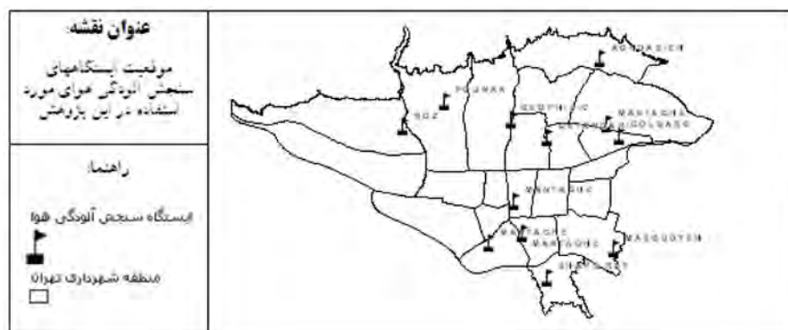
نگاره ۱: موقعیت ایستگاه‌های سنجش آلودگی هوای مورد استفاده در این پژوهش (تهیه کننده: نگارنده)
