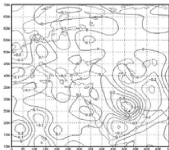
نگاره ۱۶: نقشه امگای تراز ۸۵۰ هکتوپاسکال در ساعت صفر روز ۷ ژانویه ۲۰۰۸
