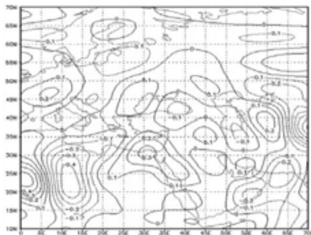
نگاره ۲۰: نقشه امگای ۸۵۰ هکتوپاسکال در ساعت صفر روز ۸ ژانویه ۲۰۰۸
