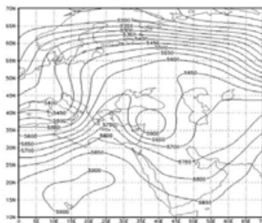
نگاره ۲۲: نقشه سطح ۵۰۰ هکتوپاسکال در ساعت صفر روز ۳۰ نوامبر ۲۰۰۹
