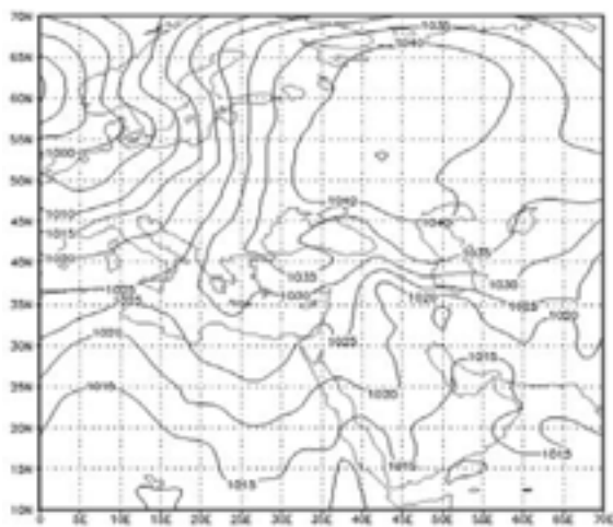
نگاره ۱۱: نقشه سطح زمین در ساعت صفر گرینویچ روز ۶ ژانویه ۲۰۰۸
