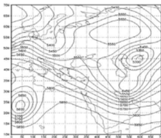
نگاره ۱۵: نقشه سطح ۵۰۰ هکتوپاسکال در ساعت صفر گرینویچ روز ۷ ژانویه ۲۰۰۸
