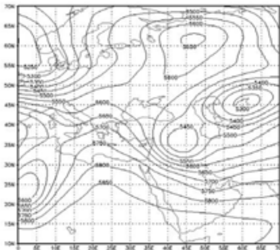
نگاره ۱۳- نقشه تراز ۵۰۰ هکتوپاسکال در ساعت صفر گرینویچ روز ۶ ژانویه ۲۰۰۸
