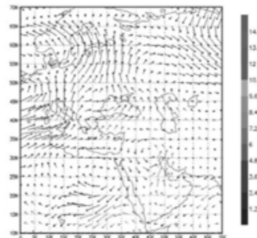
نگاره ۲۵: نقشه وزش رطوبتی سطح ۸۵۰ هکتوپاسکال در روز ۳۰ نوامبر ۲۰۰۹ (gr/kg)
