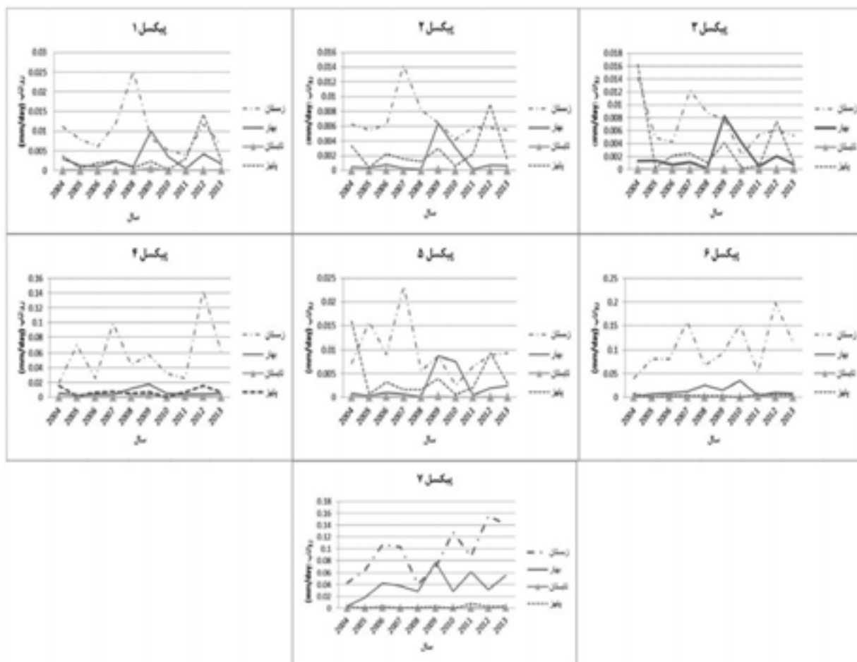
نگاره ۸: بررسی تغییرات فصلی رواناب در پیکسل‌های ۱ تا ۷ در طول سال‌های ۲۰۱۳-۲۰۰۴
