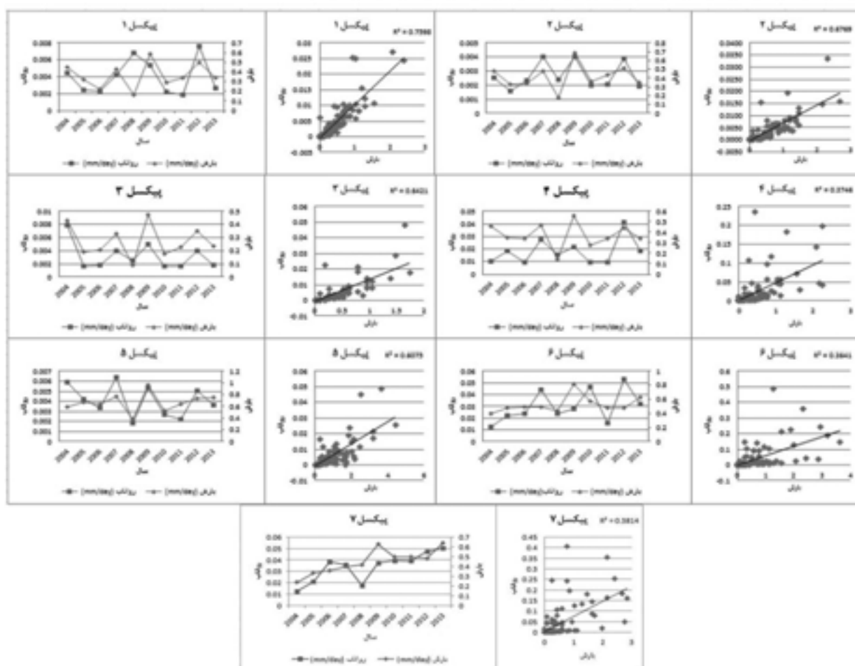
نگاره ۶: تغییرات بارش و رواناب و نمودار میزان همبستگی بارش و رواناب ماهیانه در طی ۱۰ سال برای ۷ پیکسل
