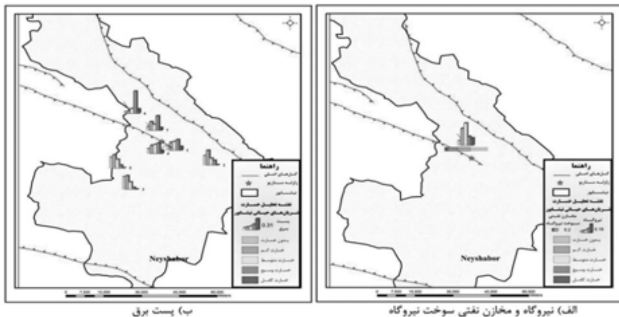
نگاره ۹: نقشه تحلیل خسارت لرزه‌ای شبکه برق به تفکیک نیروگاه و پست برق
