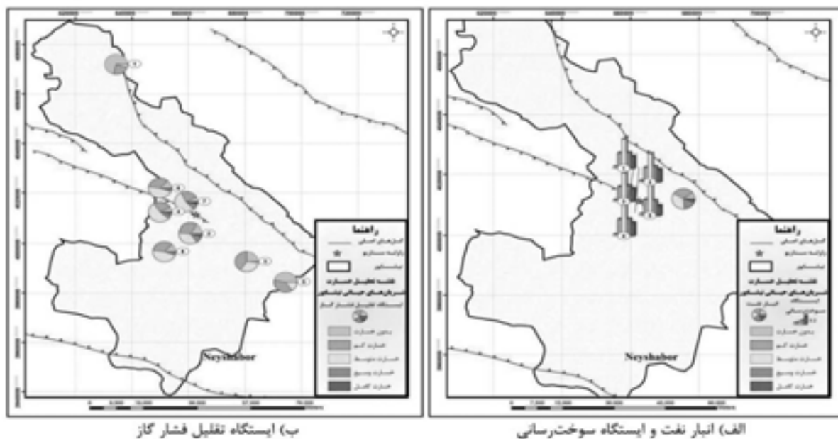
نگاره ۱۰: نقشه تحلیل خسارت لرزه‌ای شبکه سوخت به تفکیک انبار نفت، ایستگاه سوخت‌رسانی و ایستگاه تقلیل فشار گاز
