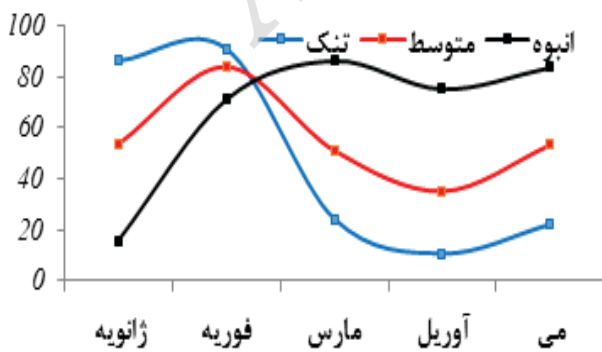
نگاره ۵: درصد نقاط دارای همبستگی منفی با شاخص NAO در ماه‌های مختلف به تفکیک هر ناحیه
