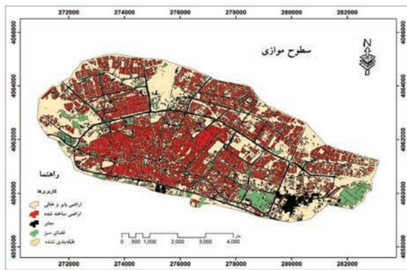
نگاره ۶: نقشه طبقه‌بندی سطوح موازی
