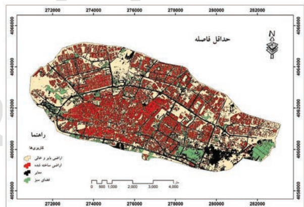
نگاره ۳: نقشه طبقه‌بندی حداقل فاصله
