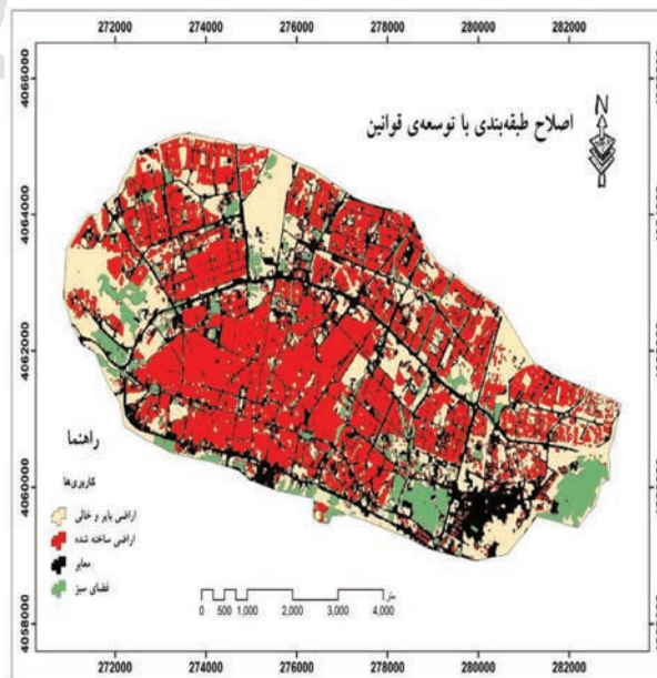
نگاره ۱۱: نتیجه طبقه‌بندی با توسعه قوانین
