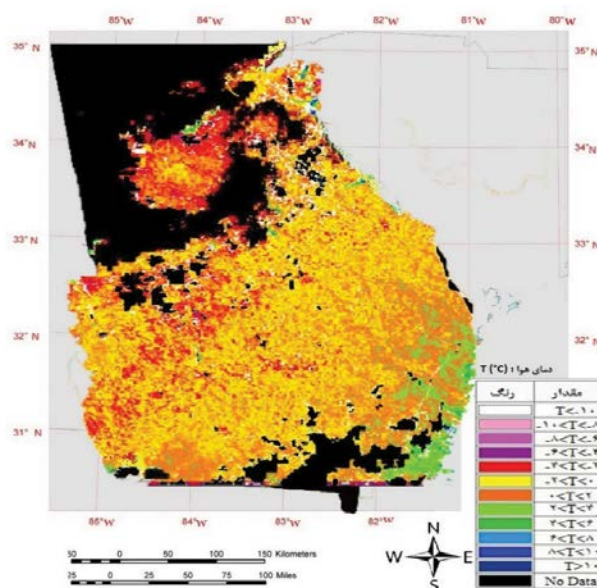
نگاره ۷: پهنه بندی دمای هوا در تاریخ ۵ دسامبر ۲۰۰۶ ساعت ۲:۱۵ بامداد
