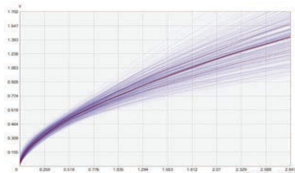
نگاره ۶: طیف وسیعی از مدل‌های سمی واریوگرام تولید
