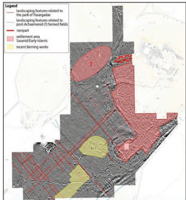
نقشه ۴: تفسیر آنومالی های مغناطیسی آشکار شده بر روی نقشه مغناطیسی، تهیه شده بین سال های ۱۳۹۴ تا ۱۳۹۶. قسمت های قرمز رنگ، ساختارهای مسکونی در جنوب تل تخت هستند.
