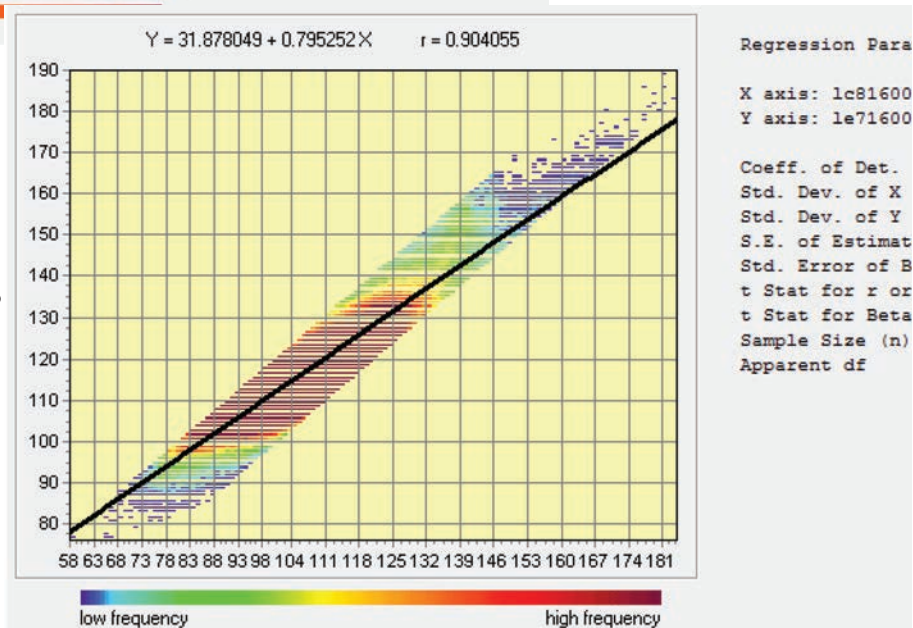
نگاره ۵: ابر پراکنش ارزش‌های پیکسلی در فضای باند قرمز برای سنجنده OLI و ETM + در مناطق همگن کاذب به همراه اطلاعات آماری خط رگرسیونی آن
