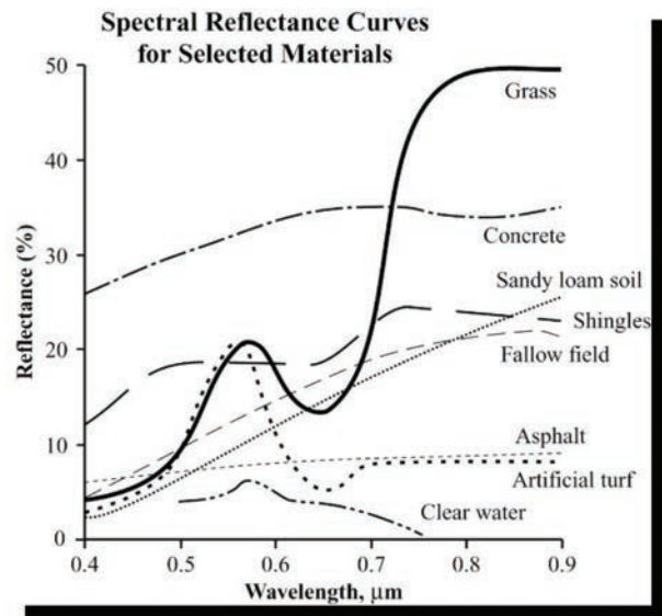
نگاره ۲: منحنی رفتار طیفی برخی از مهمترین مواد
