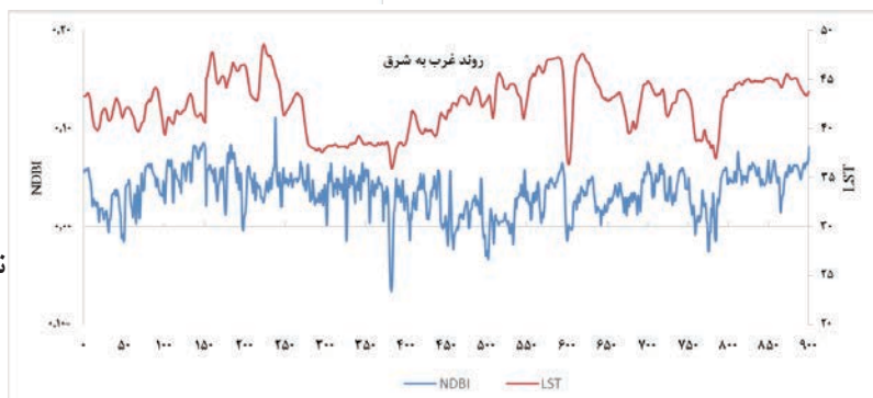
نگاره ۸: منحنی ایزوترمیک متغیرهای LST و NDBI در شرق - غرب
