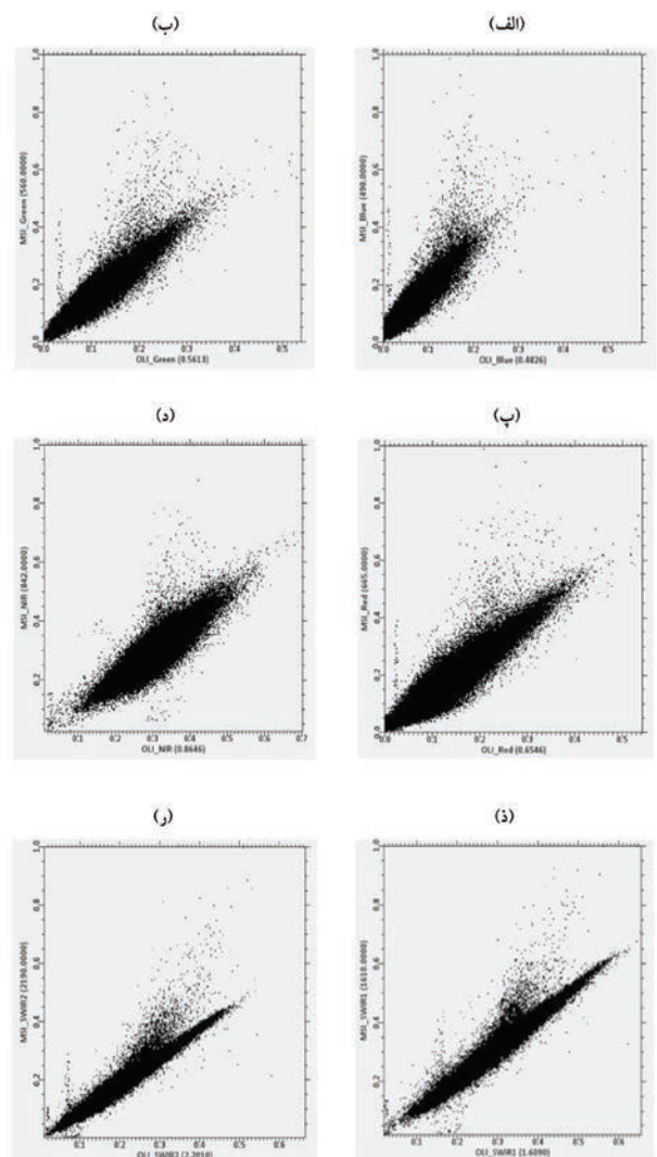
نگاره ۴: نمودار پراکنش باندهای متناظر دو سنجنده OLI و MSI مربوط به ژوئیه ۲۰۱۸، (الف) باندهای آبی، (ب) سبز، (پ) قرمز، (د) مادون قرمز نزدیک، (ذ) مادون قرمز طول موج کوتاه ۱، (ر) مادون قرمز طول موج کوتاه ۲.
