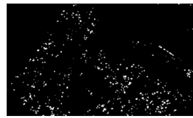
قطبش VV
