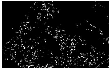
قطبش VH
