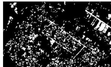
باند SWIR
