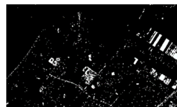
شاخص ARVI
