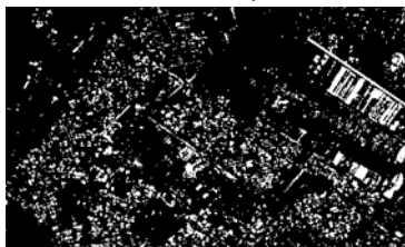
باند NIR
