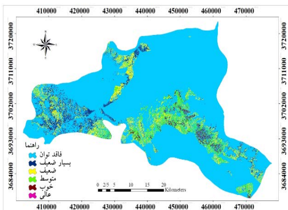
نگاره ۱۱: نقشه طبقه‌بندی توان منطقه برای استقرار شهرک صنعتی با روش ترکیب خطی وزنی
