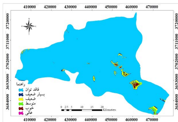
نگاره ۵: نقشه طبقه‌بندی توان منطقه برای استقرار شهرک صنعتی با روش روی هم‌گذاری فازی
