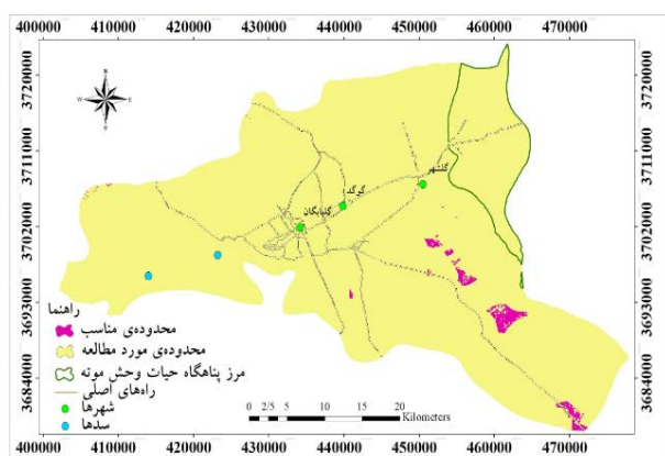
نگاره ۶: نقشه تلفیق طبقات توان متوسط تا عالی منطقه برای استقرار شهرک صنعتی با روش روی هم‌گذاری فازی
