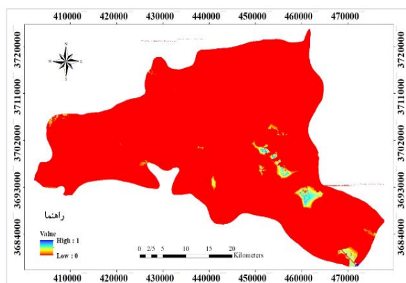
نگاره ۴: نقشه توان منطقه برای استقرار شهرک صنعتی با روش روی هم‌گذاری فازی
