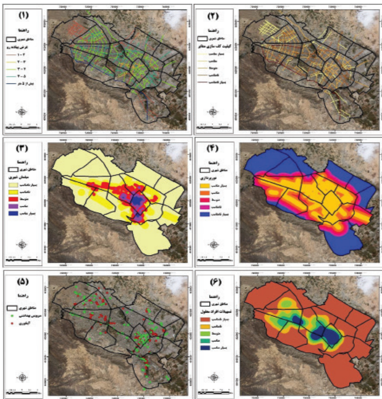
نگاره ۴: (۱) عرض پیاده‌رو (۲) کیفیت کف‌سازی (۳) میلان شهری (۴) نورپردازی (۵) سرویس بهداشتی و آبخوری (۶) تسهیلات افراد معلول
