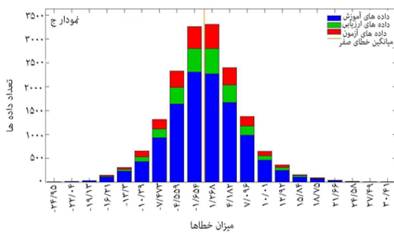
نگاره ۳: نمودار هیستوگرام مقادیر خطاها برای روش‌های پیش‌رونده (الف)، پس‌رونده (ب)، نمایه کاهش درصدی (ج) و گام به گام (د)
