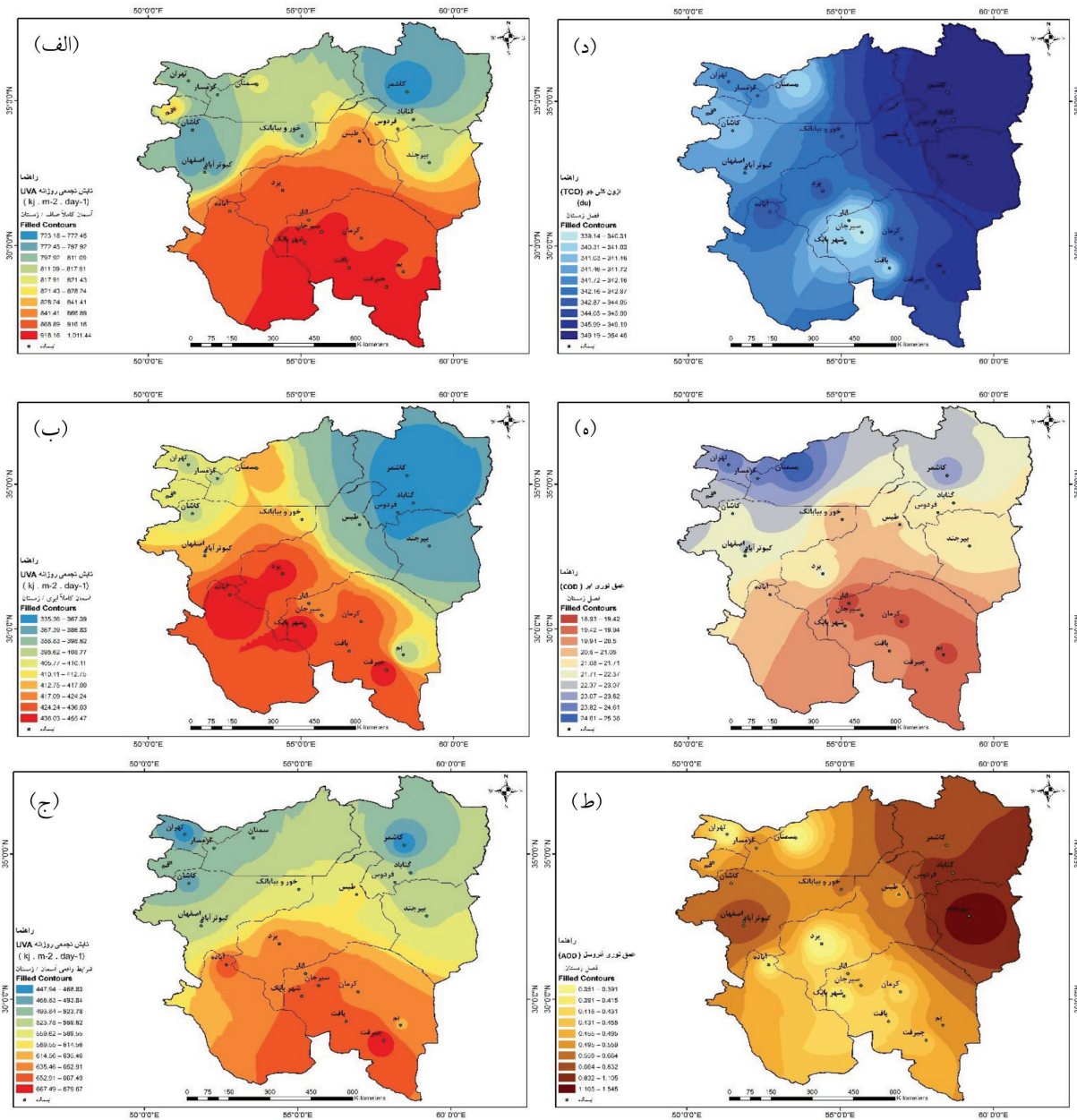
نگاره ۵: میانگین ۱۳ ساله تابش جمعی روزانه UVA (کیلوژول بر متر مربع در روز): الف) آسمان کاملاً صاف، ب) آسمان کاملاً ابری، ج) آسمان واقعی د) ازون کلی جو (دایسون)، ه) عمق نوری ابر، ط) عمق نوری آتروسول در فصل زمستان
