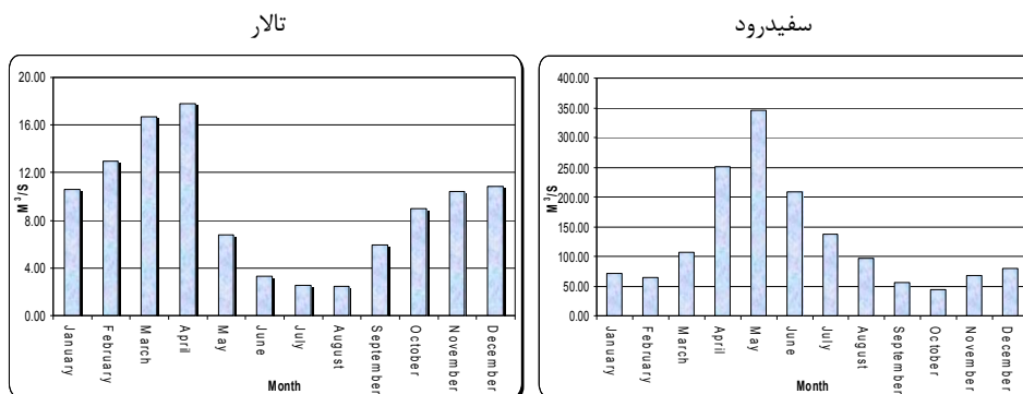
شکل ۲- نمونه‌ای از رژیم ماهانه آبدهی رودخانه حوضه ایرانی خزر (۲۰۰۶-۱۹۸۳)
