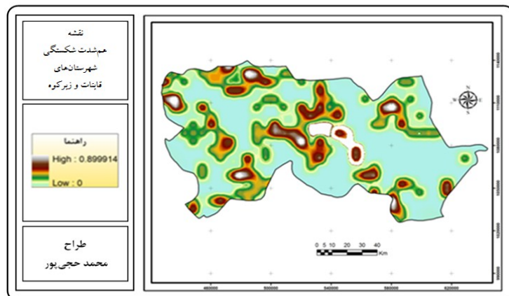
شکل ۴. نقشه هم‌شدت شکستگی شهرستان‌های قاینات و زیرکوه
