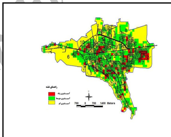
شکل ۱۴- نقشه نهایی آسیب پذیری برحسب زون بندی شهر گرگان
