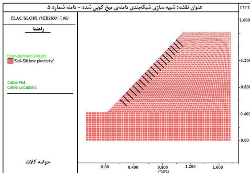
شکل ۱۱- شبیه‌سازی شبکه‌بندی دامنه میخ‌کوبی شده در دامنه ۵.
