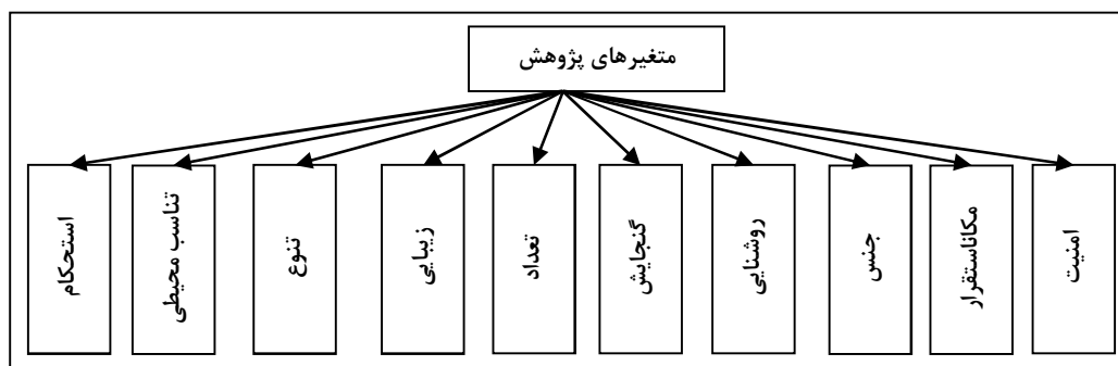
شکل ۱: متغیرهای پژوهش
