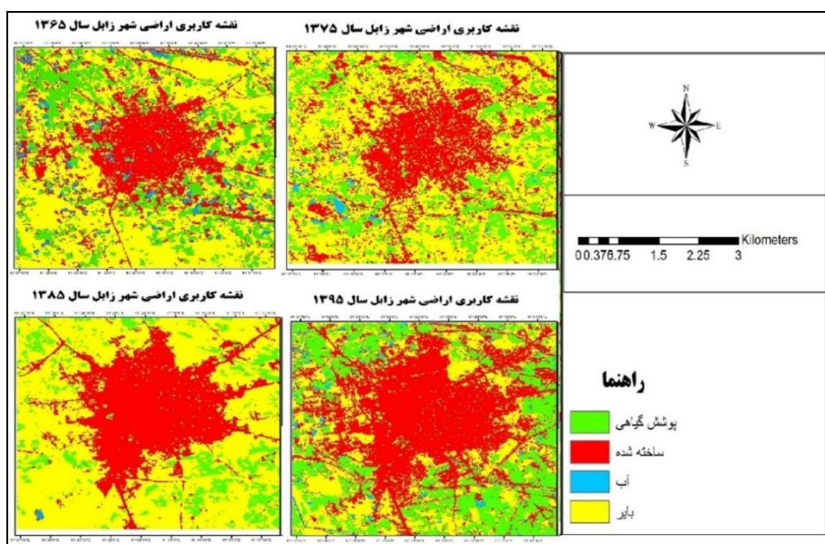
شکل ۲: نقشه‌های طبقه‌بندی کاربری اراضی سال‌های ۱۳۶۵_۱۳۷۵_۱۳۸۵_۱۳۹۵ (منبع: نگارندگان، ۱۳۹۷)
