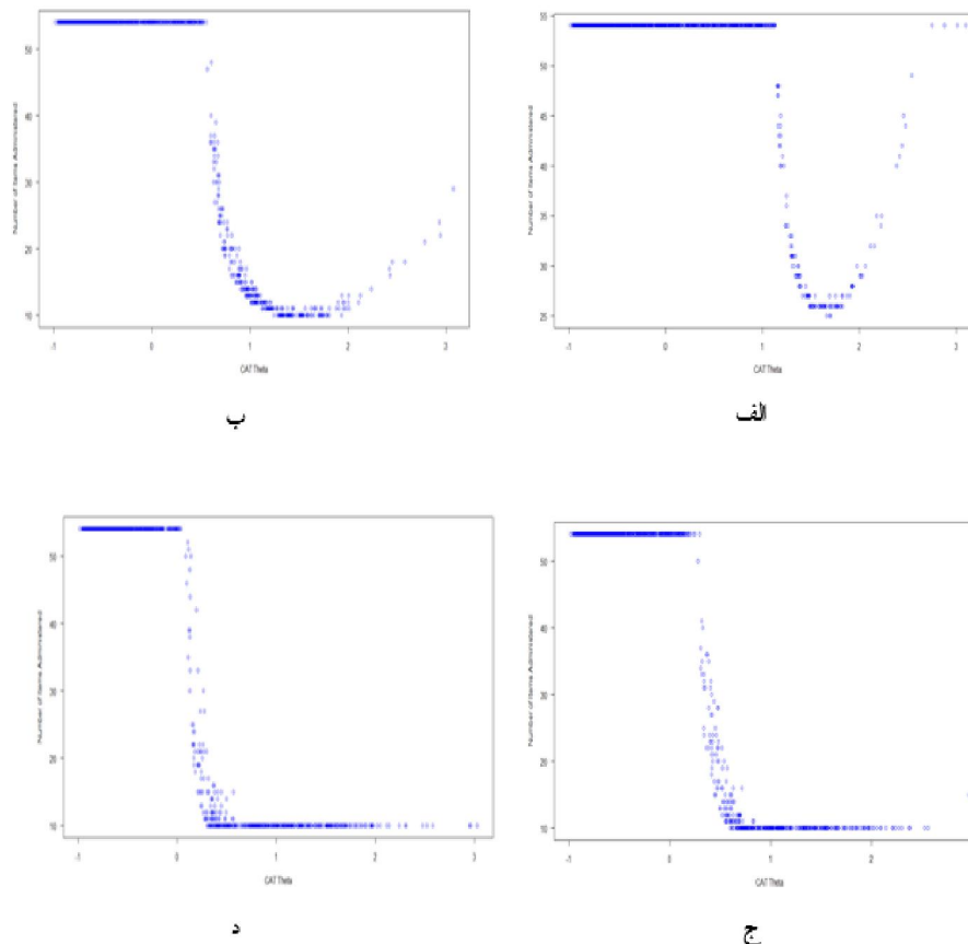
شکل (۲) تعداد سؤال‌های اجرا شده در روش برآورد پسین مورد انتظار: الف) ملاک خاتمه خطای استاندارد ثابت ۰/۲ (ب) ملاک خاتمه خطای استاندارد ثابت ۰/۳ (ج) ملاک خاتمه خطای استاندارد ثابت ۰/۴ (د) ملاک خاتمه خطای استاندارد ثابت ۰/۵
