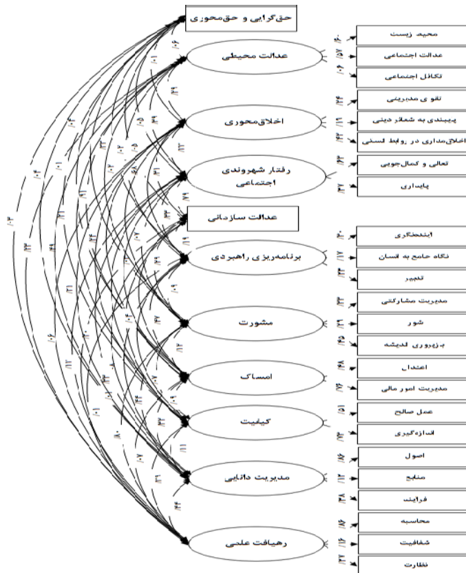
شکل ۲: ساختار عاملی سنجی عقلانیت در سازمان از دیدگاه اسلام Fig. 2: Factor Structure of Rationality Measure from Islam View
