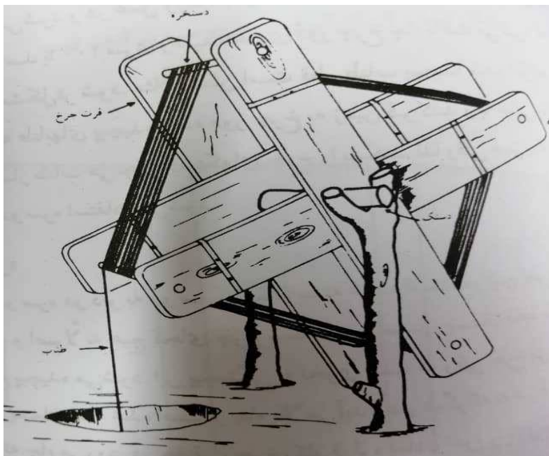
عکس ۲- چرخ چاه
